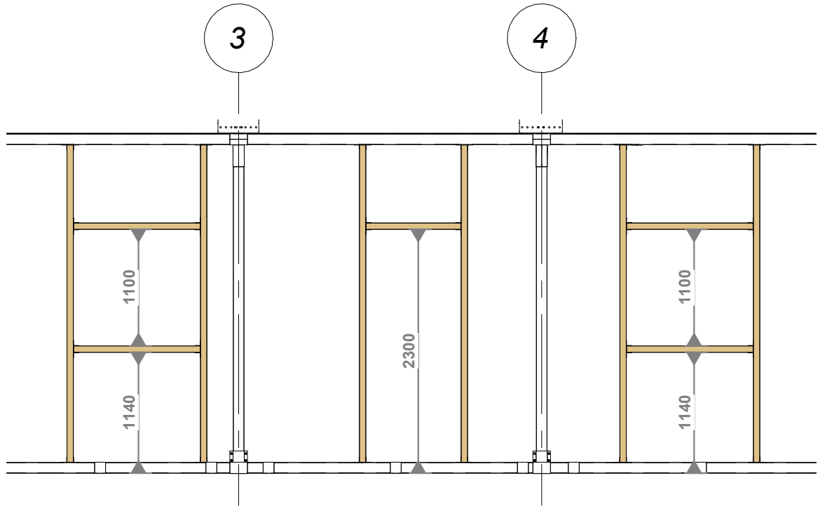
2 Detalle Altura 1 T-08 1 : 50
