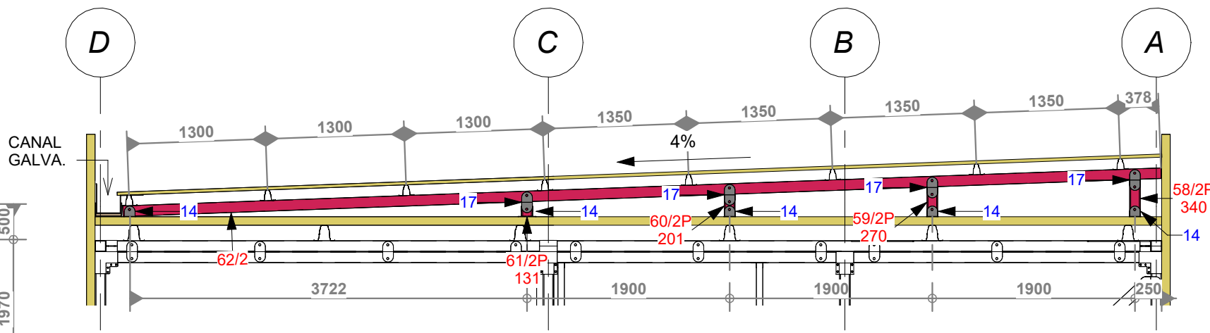
2 Sección 9 T-09 1 : 50
