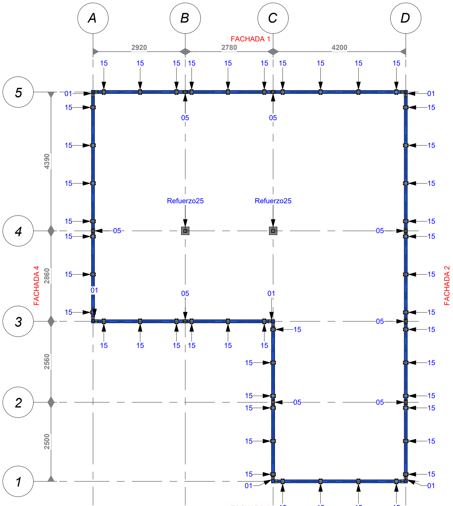
1 Uniones Anillo Inferior U-01 1 : 75
