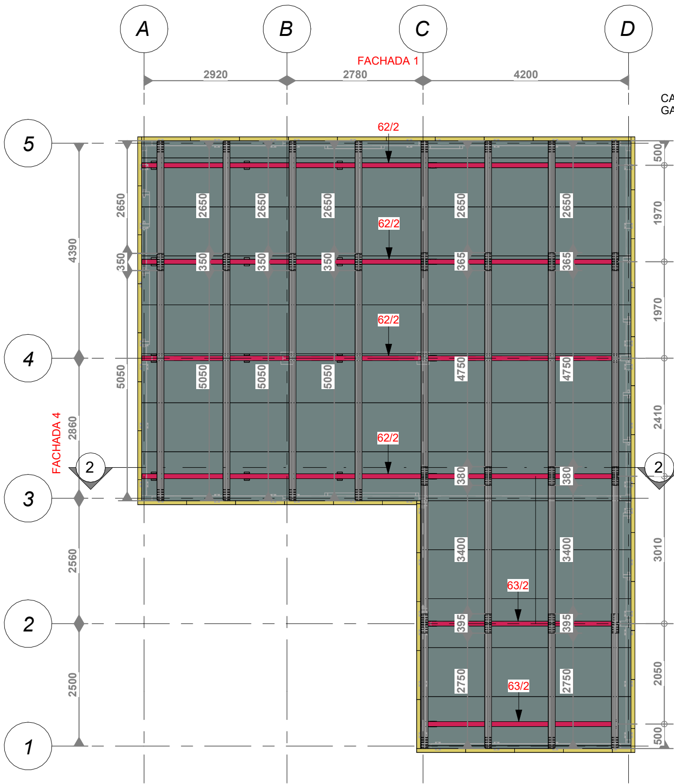
1 Subestructura T-09 1 : 75
