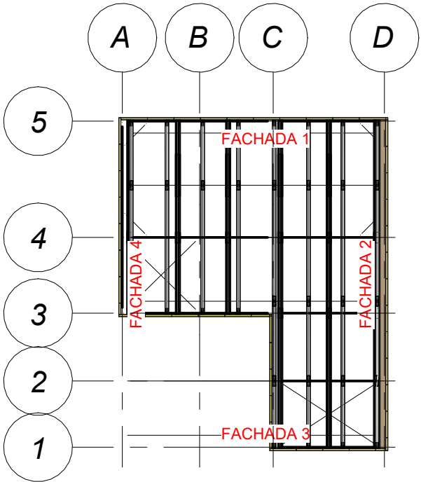
3 Referencia 1 P-03 1 : 200
