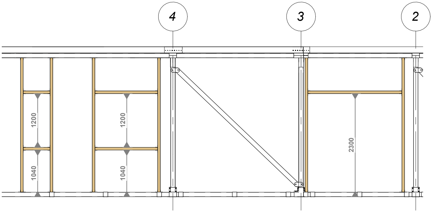
4 Detalle Altura 3 T-08 1 : 50
