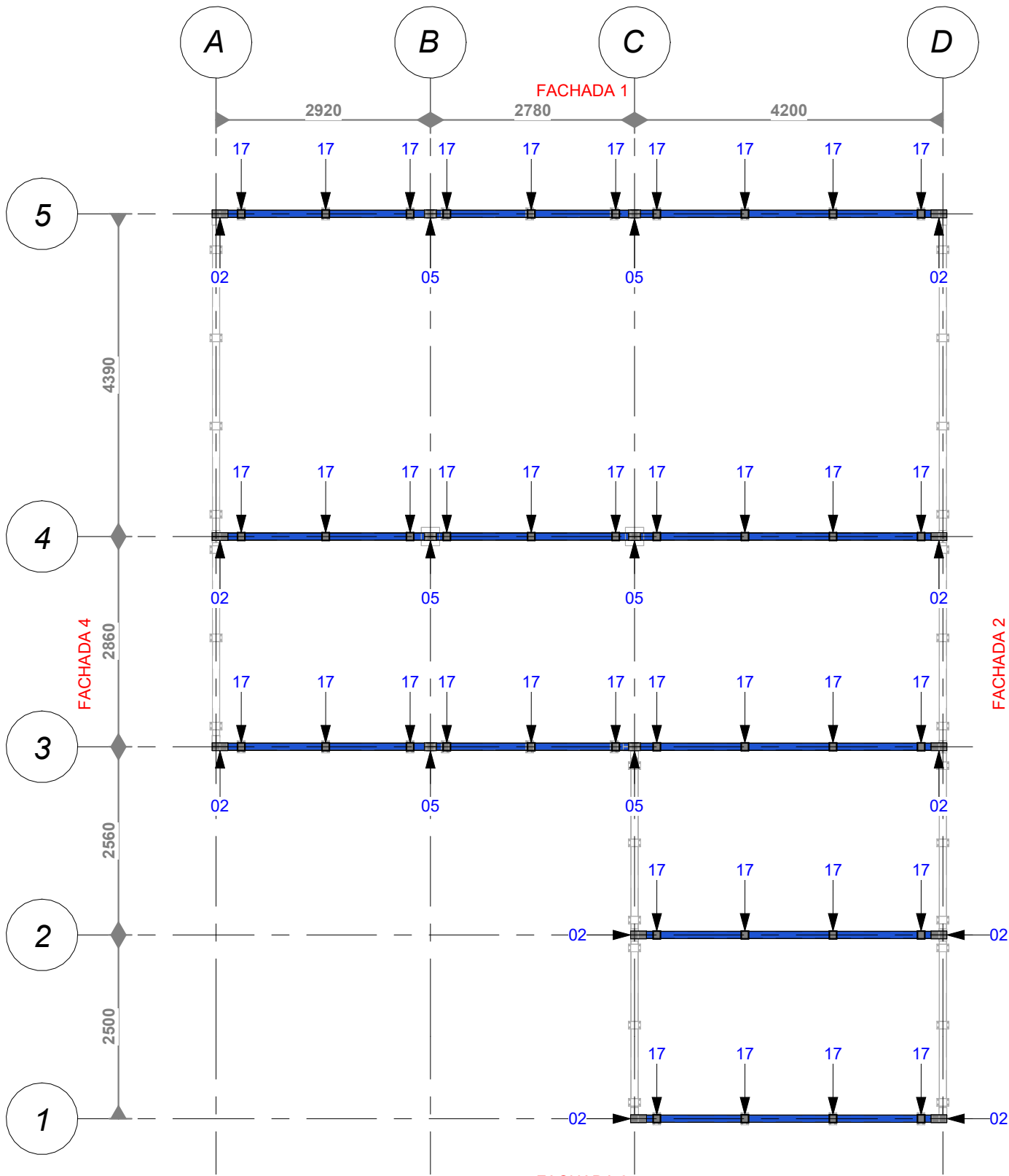
1 PB Uniones 1 U-02 1 : 75
