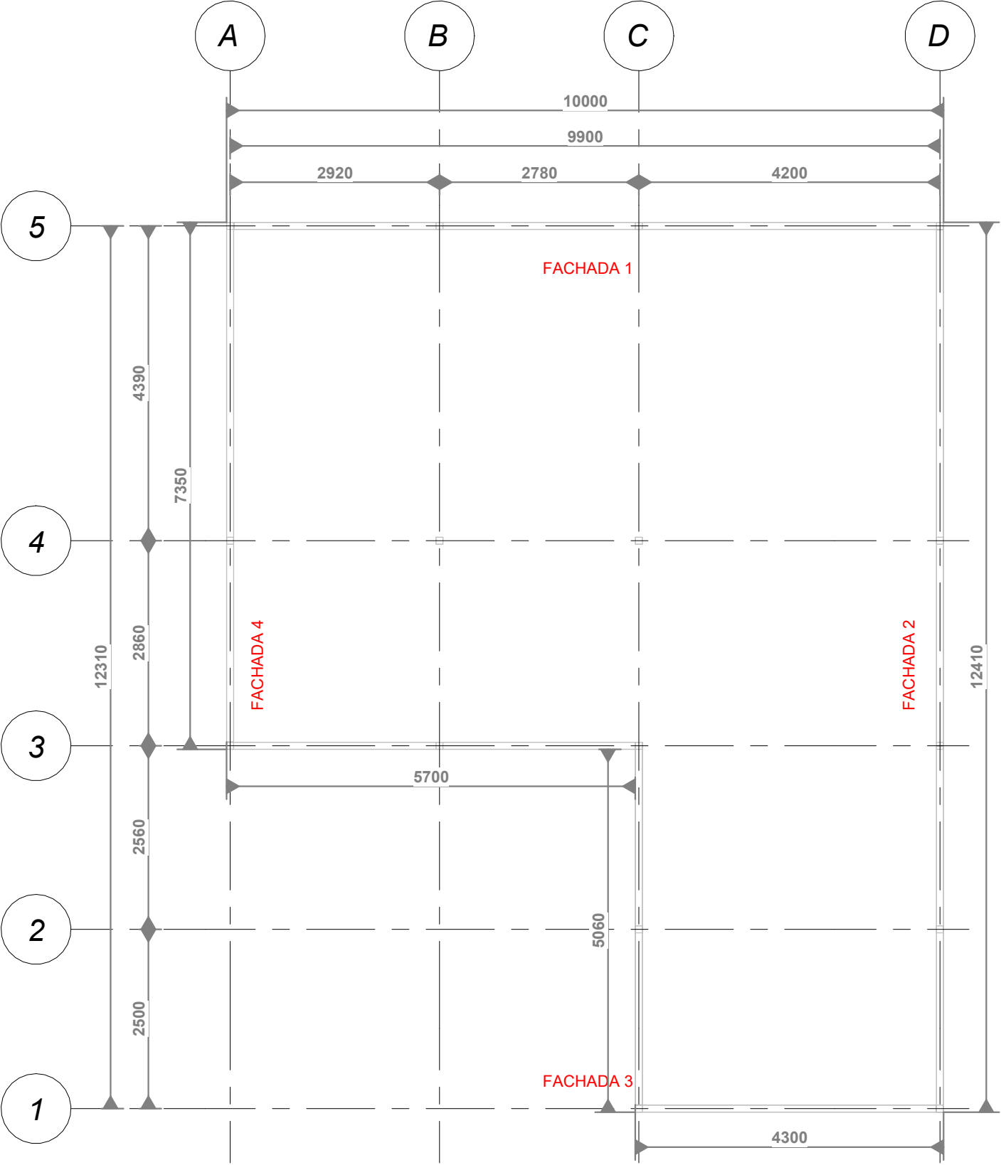
1 Replanteo T-00 1 : 75
