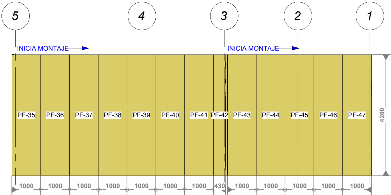
1 Fachada 4 P-06 1 : 75
