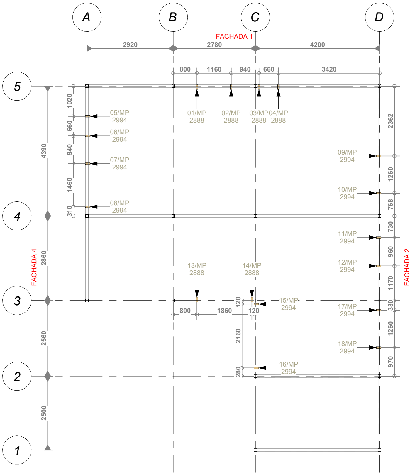
1 Pilares premarcos T-06 1 : 75
