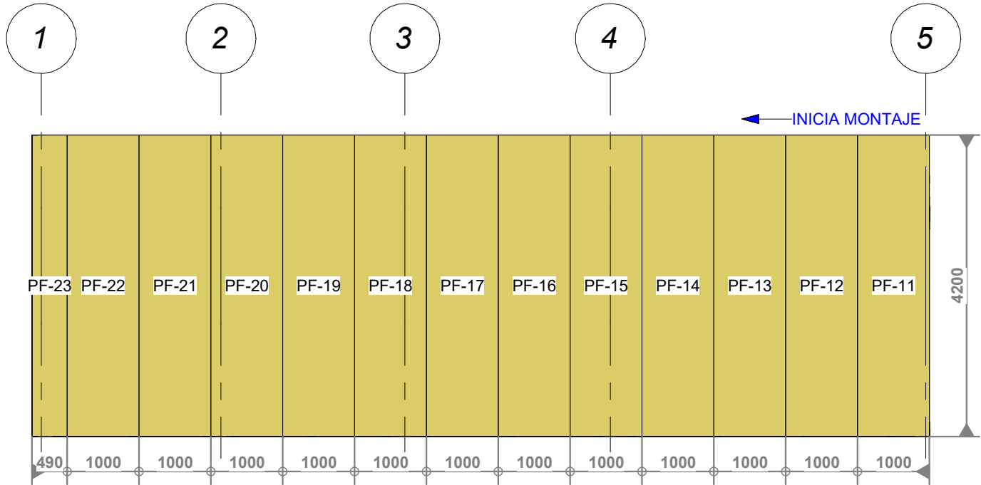
1 Fachada 2 P-04 1 : 75
