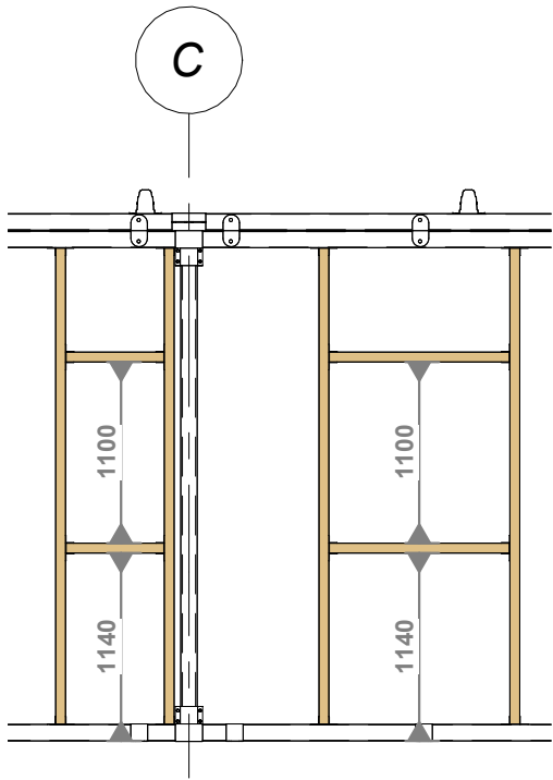
1 Detalle Altura T-08 1 : 50
