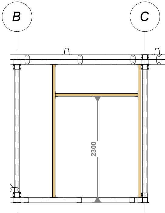
3 Detalle Altura 2 T-08 1 : 50
