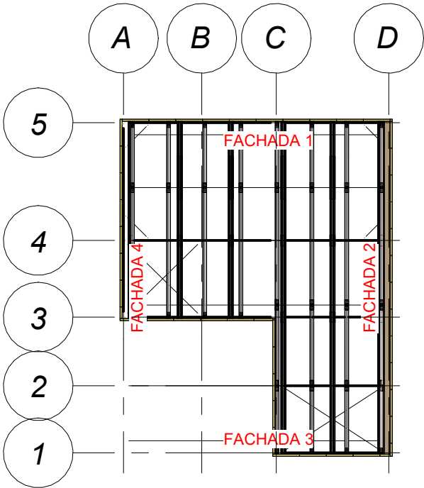
3 Referencia 4 P-06 1 : 200
