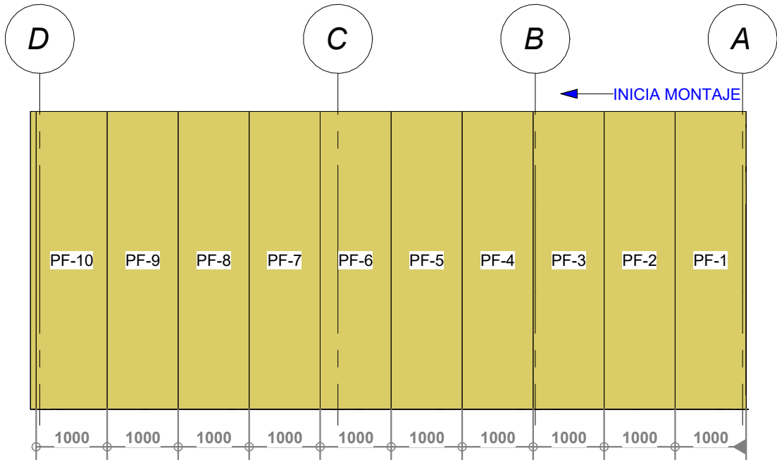
1 Fachada 1 P-03 1 : 75
